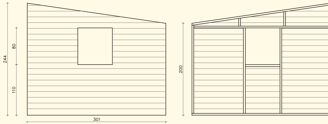
Panel frontal derecho
