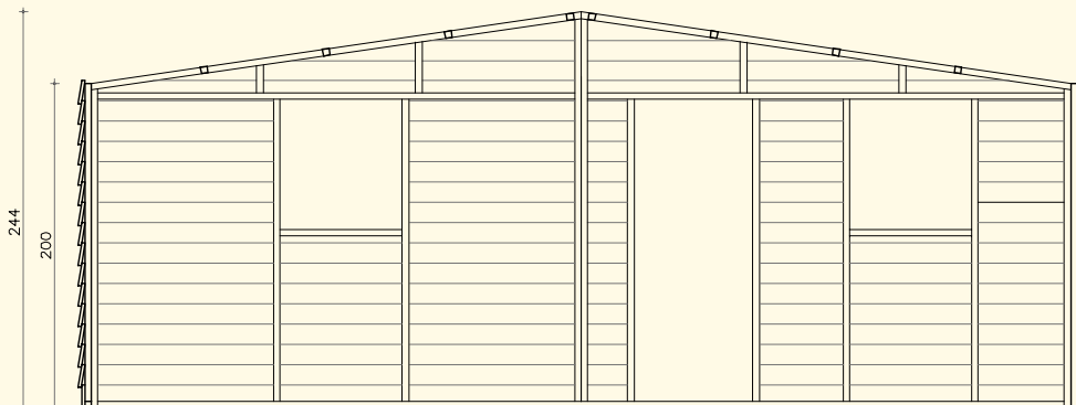
Corte longitudinal El modelo actual
