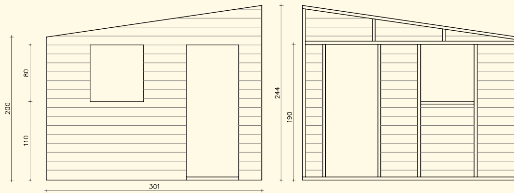
Panel frontal izquierdo
