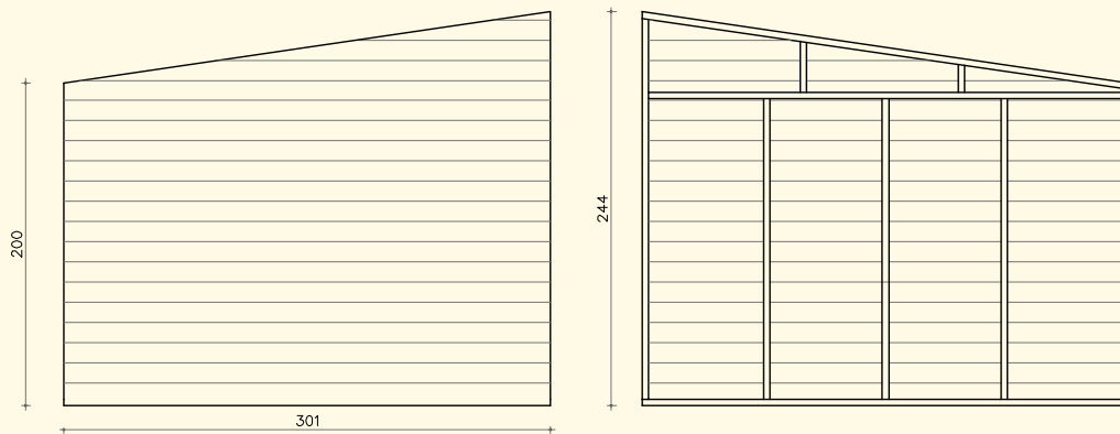
Panel posterior izquierdo
