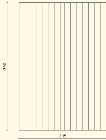
Panel de piso El modelo actual
